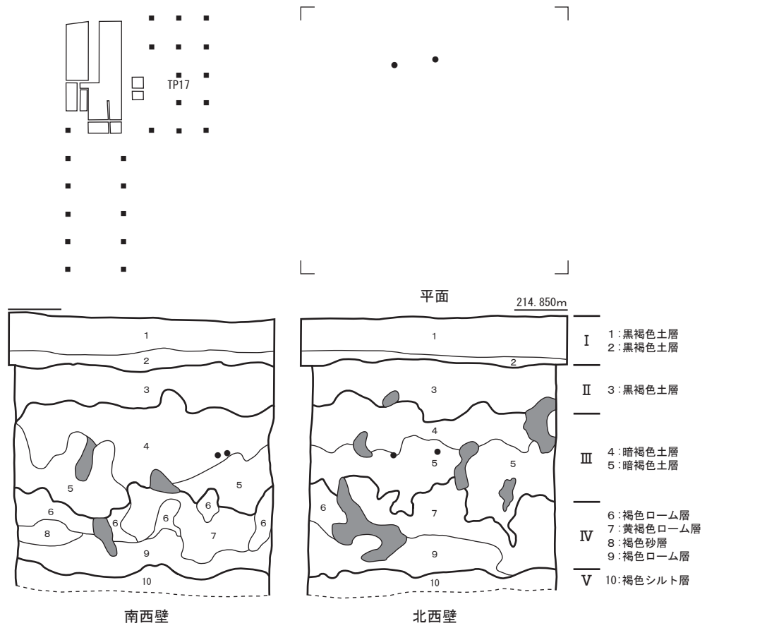
第38図 TP17土層断面図・遺物分布図 (S=1/20)
