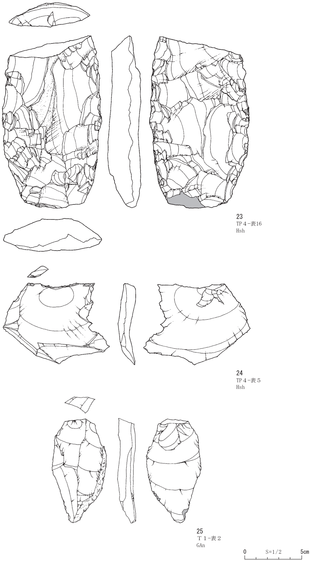
第56図 石器実測図 4 両面調整石器・剥片(2 b)・剥片(2 c)
