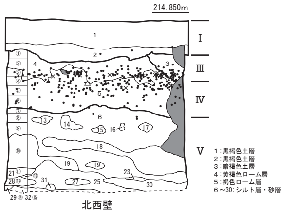
TP 1 土層断面図 (S=1/20)
